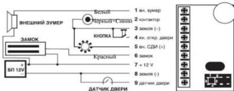
схема подключения контроллера
